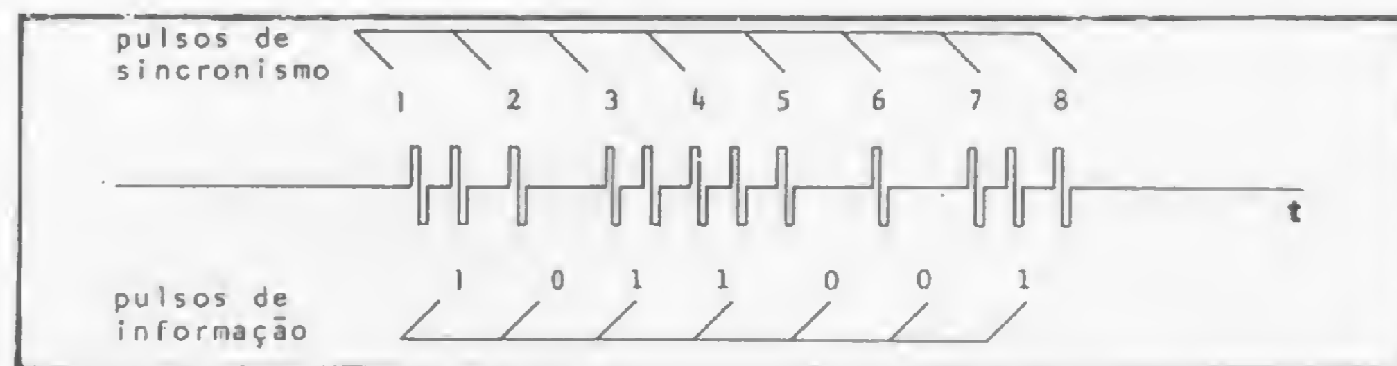
Figura 1 — Forma de onda.
